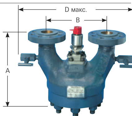
Предохранительный клапан переключатель с одним активным устройством
